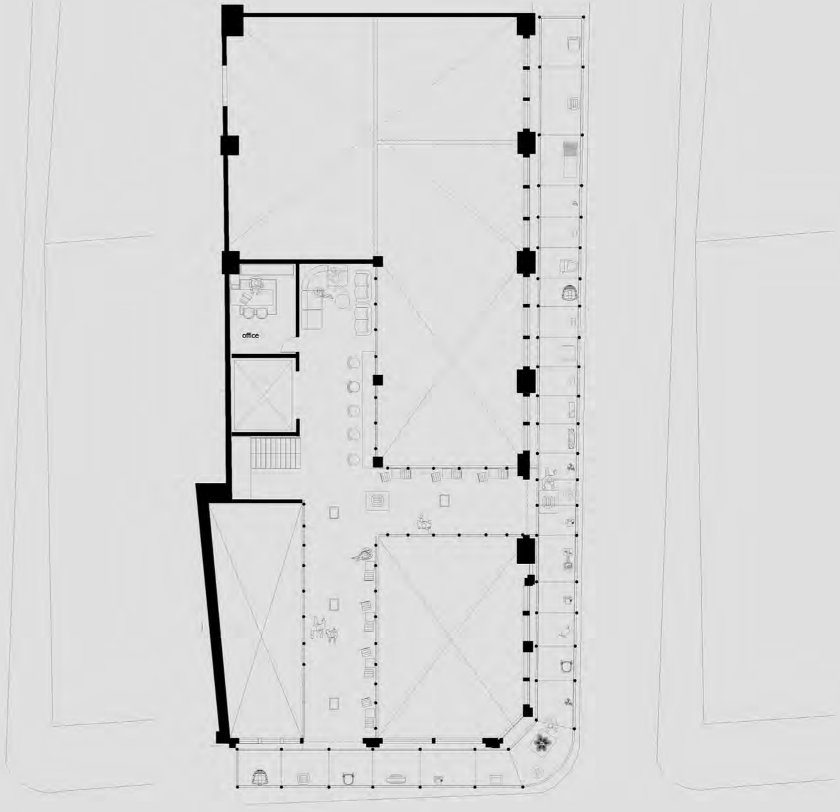
F1 PLAN 1:100
